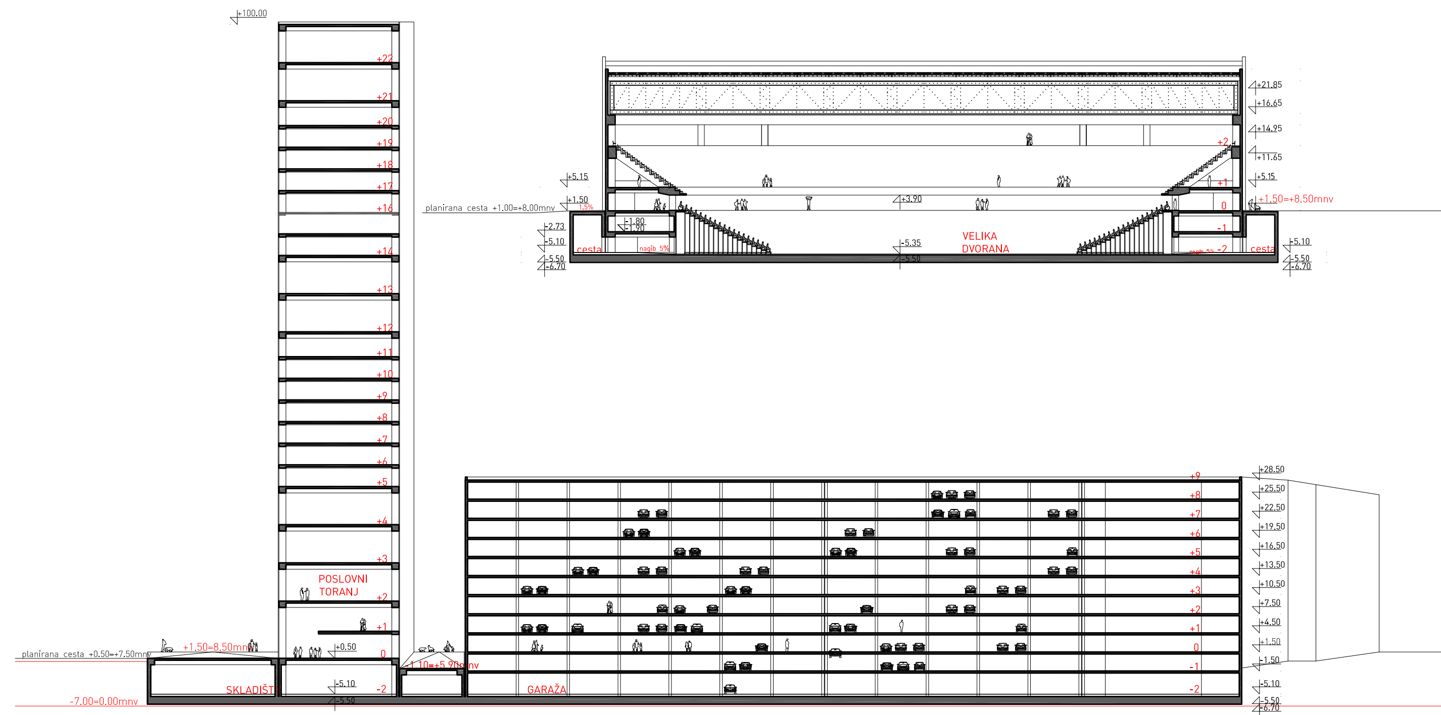
PRESJEK C - C
